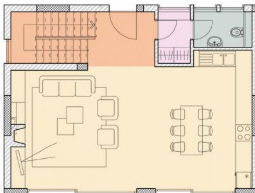
КЪЩА БЗ РЗП - 229.5m 2
